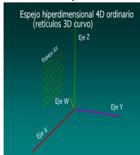
Ilustración 102: Espejo hiperdimensional en un universo 4D ordinario
