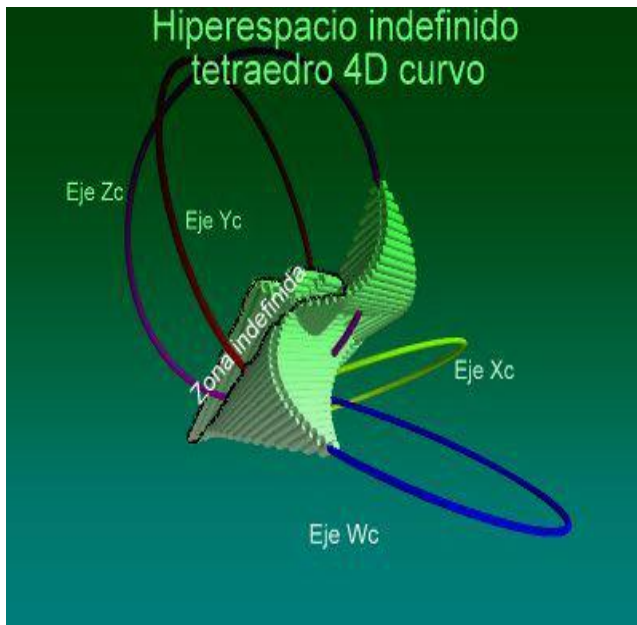
Ilustración 100: Zona de Heisemberg o zona de paso a dos mundos o realidades
