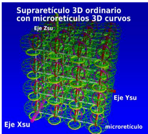
Ilustración 101: Supraretículo 3D ordinario con microretículos 3D curvos
